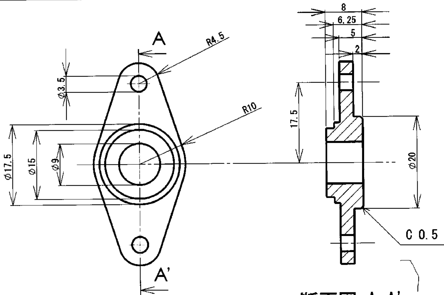
断面図 A-A'
