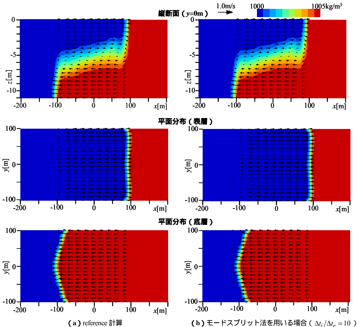
図-4 縦断面及び平面（表・底層）における密度フロントの瞬間像（ t=360s ）
