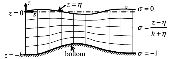
(b) 鉛直座標系
