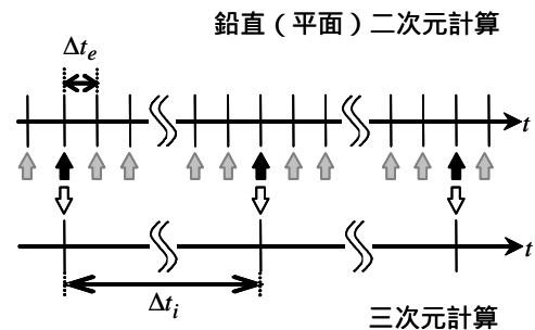
図-1 本モードスプリット法における計算時間間隔の設定
