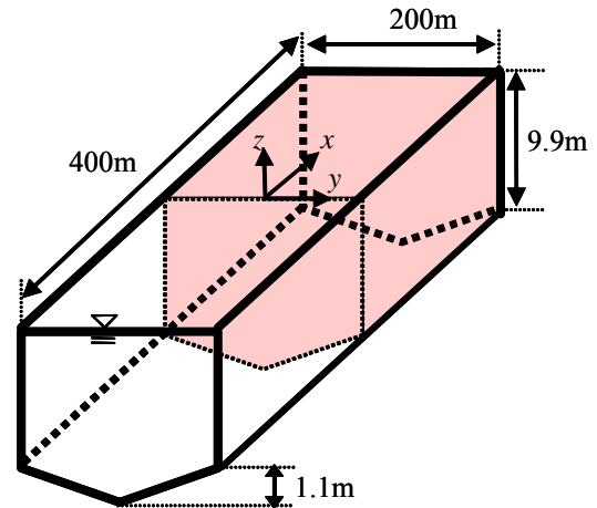
図 - 3 計算領域の設定
