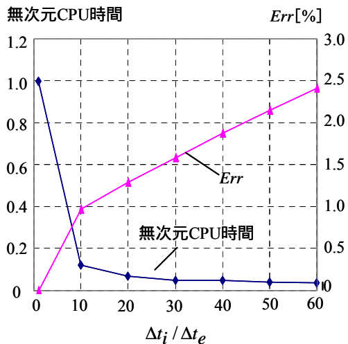
図-6 無次元 CPU 時間と計算誤差 Err(t=360s)
