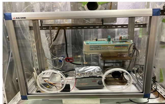
静電噴霧装置
