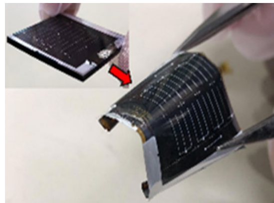
試作したCIGSフレキシブル太陽電池
